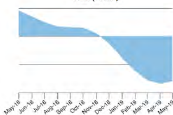
TRIX (13 mo)
