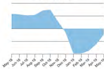
MACD (13 mo)
