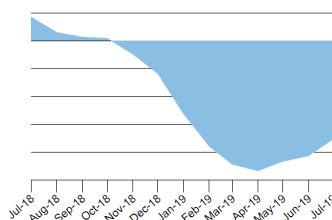
TRIX (13 mo)
