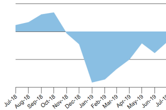
MACD (13 mo)
