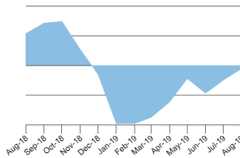
MACD (13 mo)
